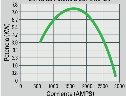
Curva de Potencia 39PE de 12V
